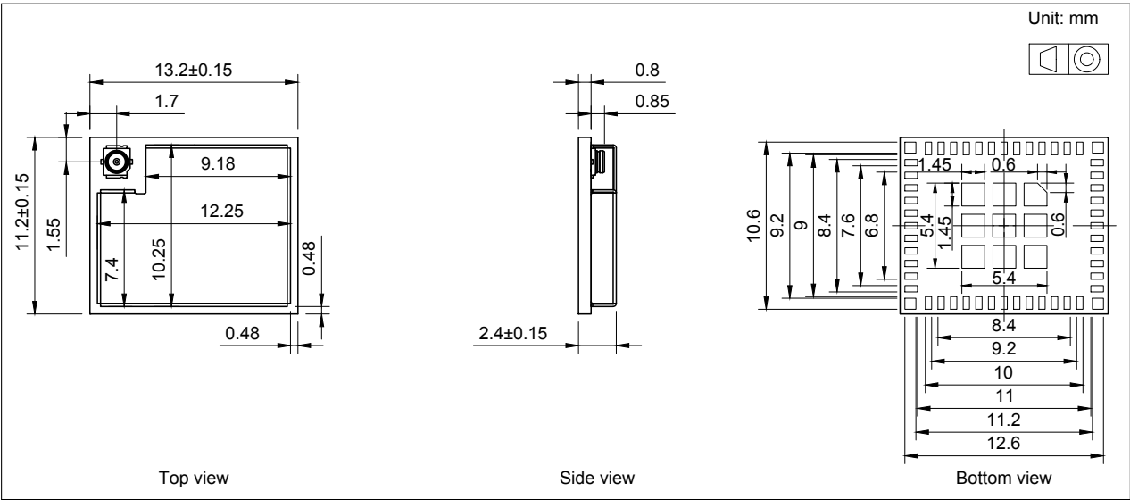
图 11: ESP32-PICO-MINI-02U 模组尺寸
