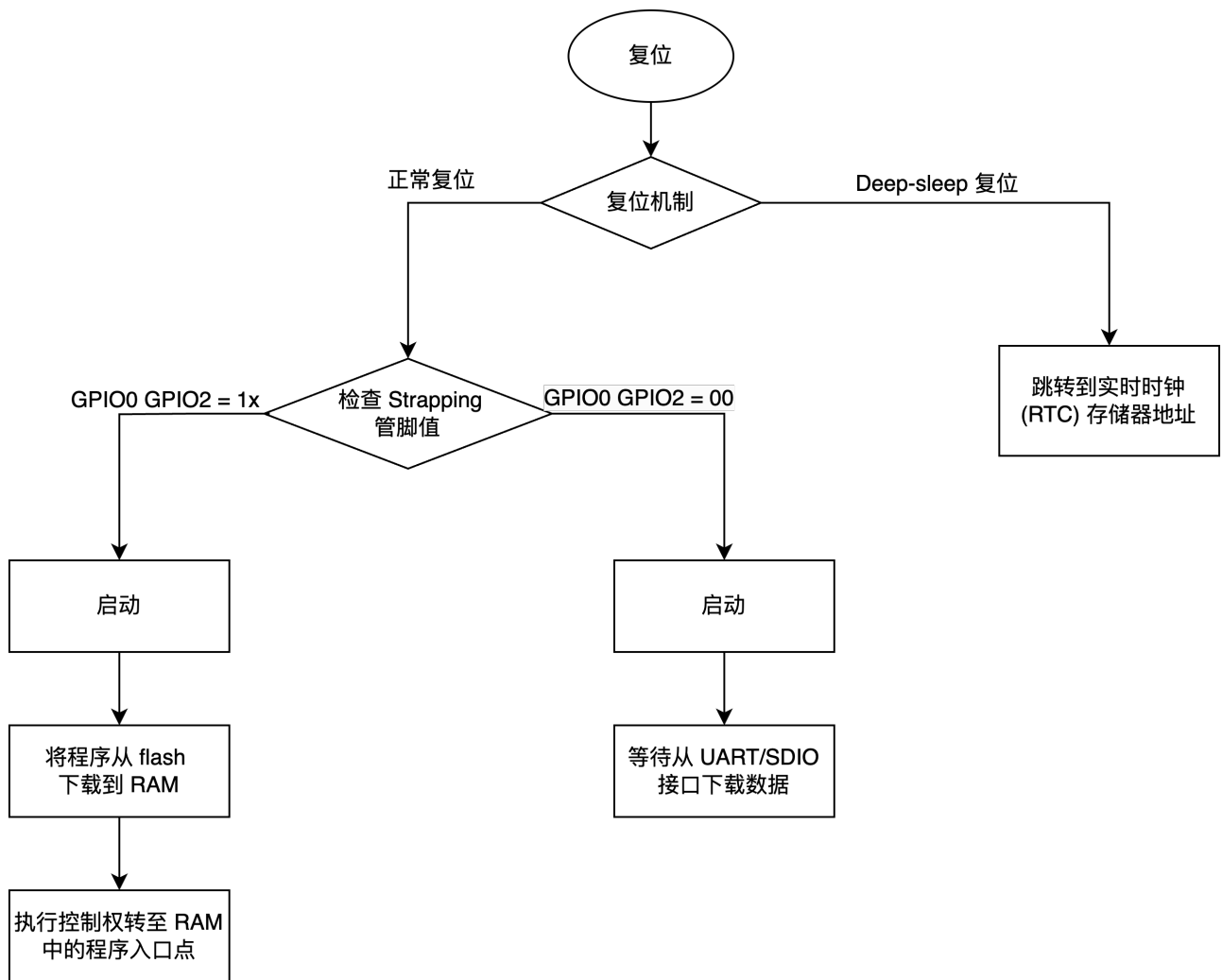
图 6: 芯片启动流程
