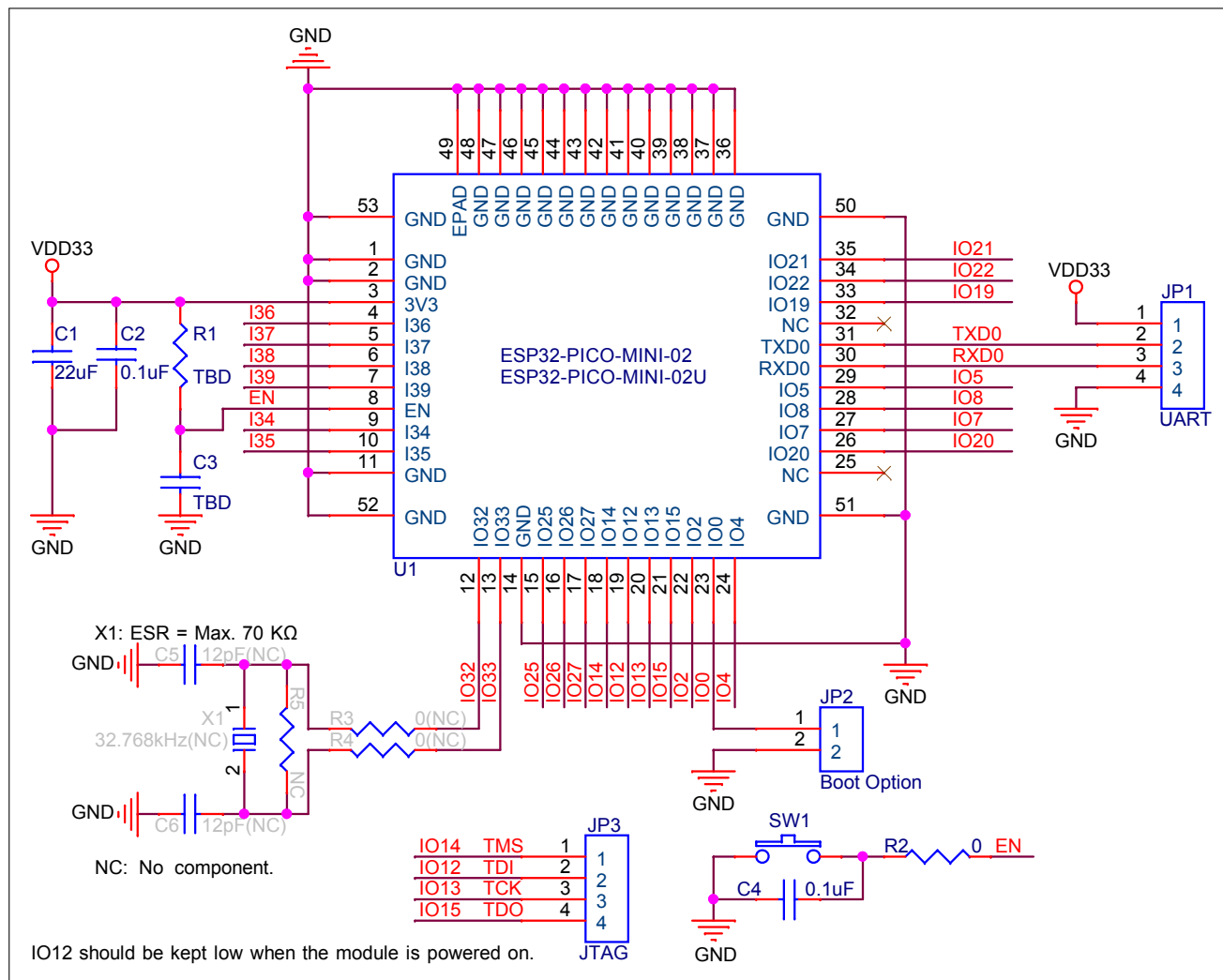
图 9: 外围设计原理图
