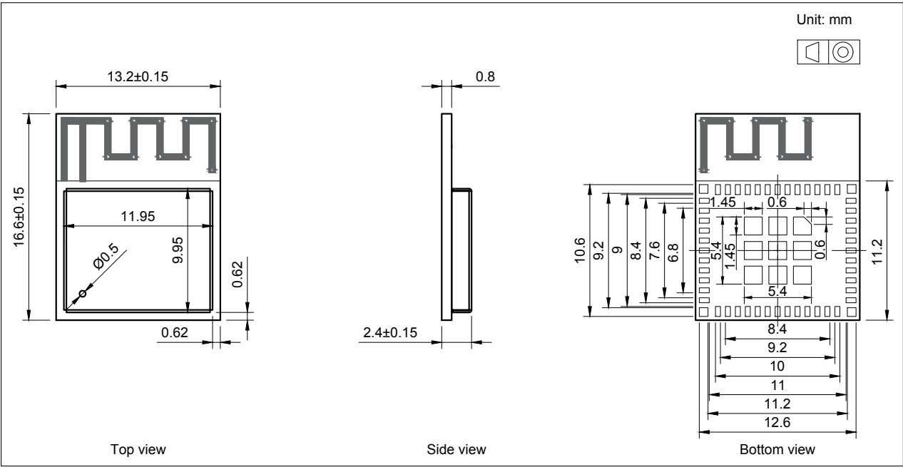
图 10: ESP32-PICO-MINI-02 模组尺寸
