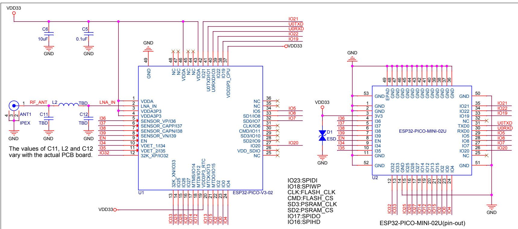
图 8: ESP32-PICO-MINI-02U 原理图
