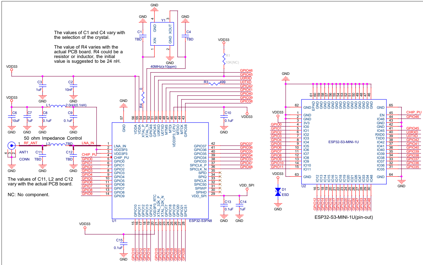
图 6: ESP32-S3-MINI-1U 原理图
