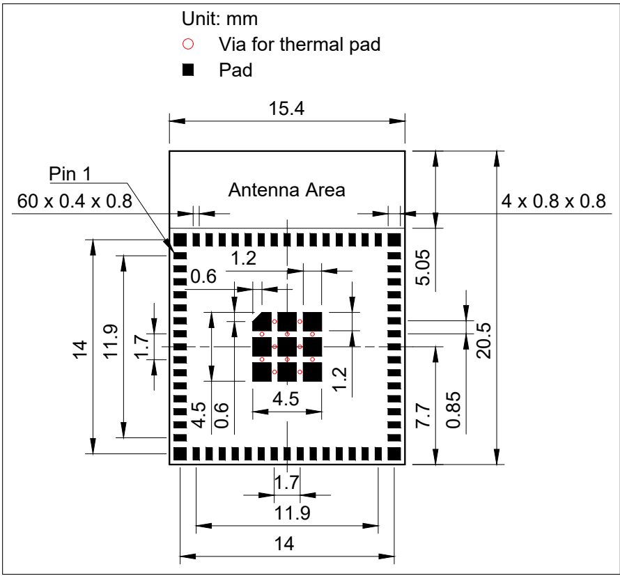
图 11: ESP32-S3-MINI-1 推荐 PCB 封装图
