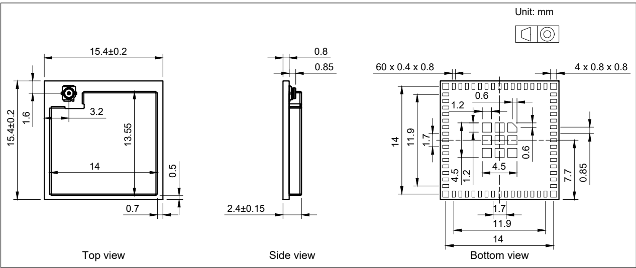
图 9: ESP32-S3-MINI-1U 模组尺寸
