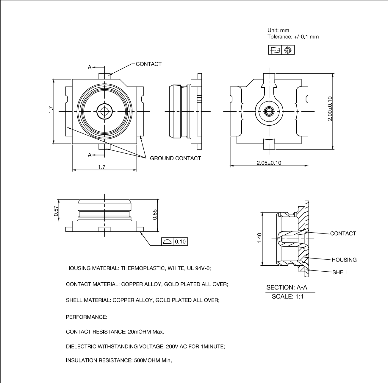
图 10: 外部天线连接器尺寸图
