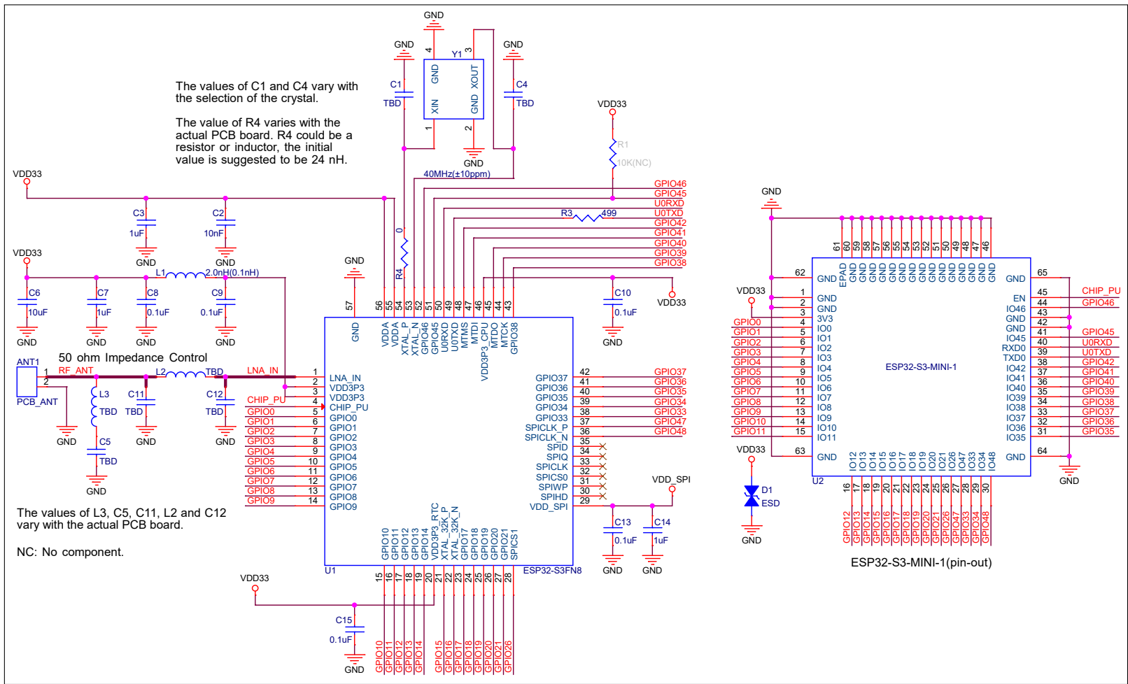
图 5: ESP32-S3-MINI-1 原理图
